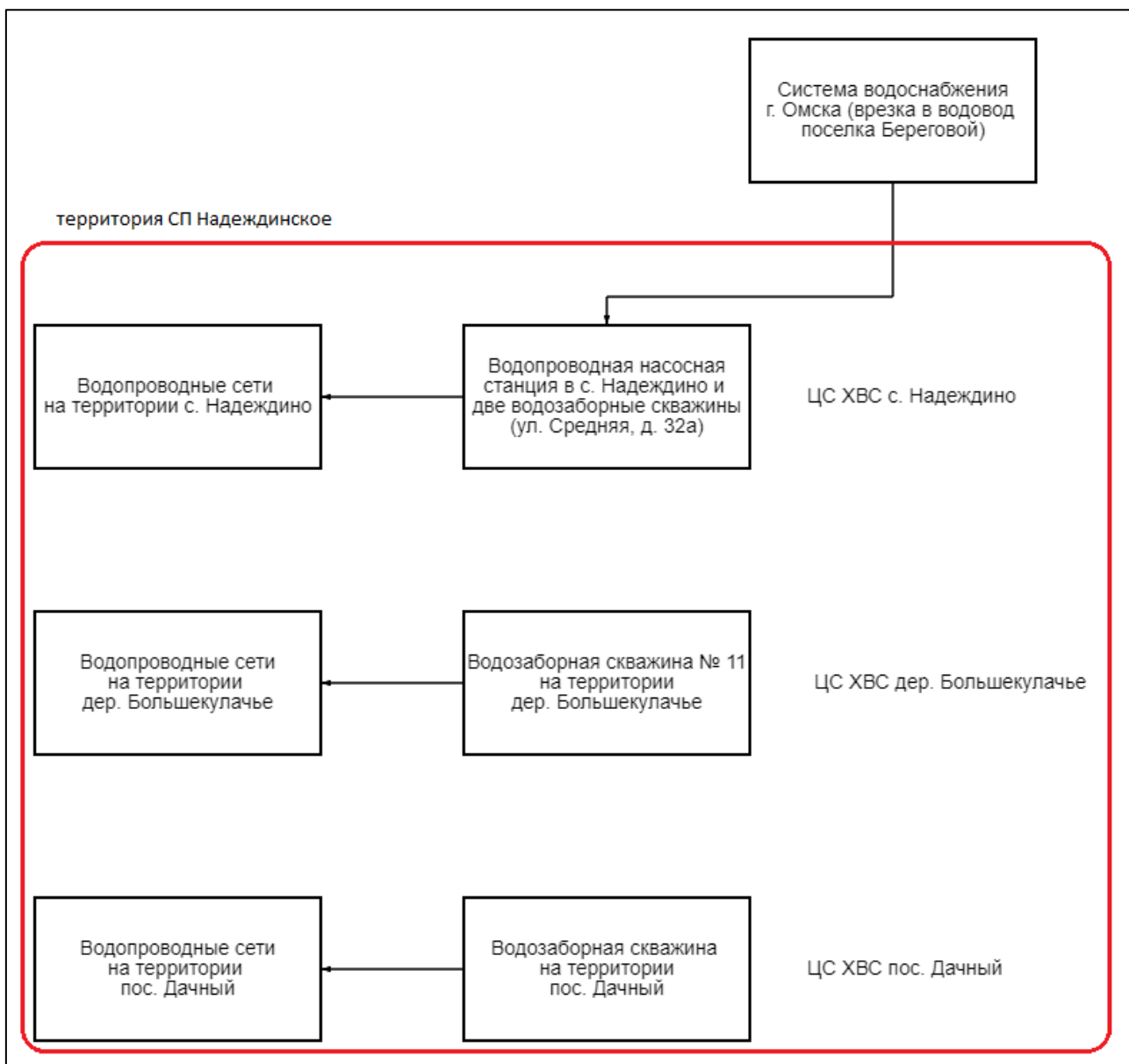
Рисунок 1.1.1 – Структурная схема централизованного водоснабжения СП Надеждинское
